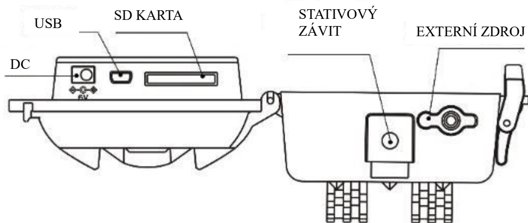
Obr. 2: Pohled spodní
